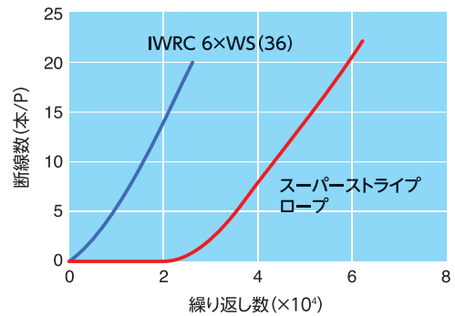
● 疲労試験結果 (D/d=16、安全率=6、U曲げ)
